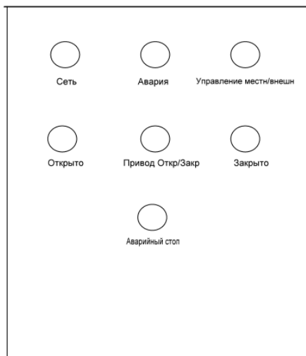
Модель ШУЭП-9 001.000.380
